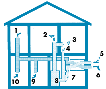
Système de ventilation avec VRC
