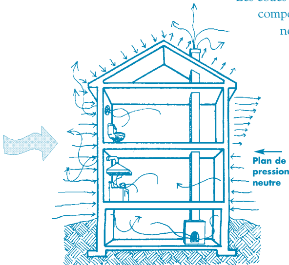
Forces qui causent les fuites d'air
